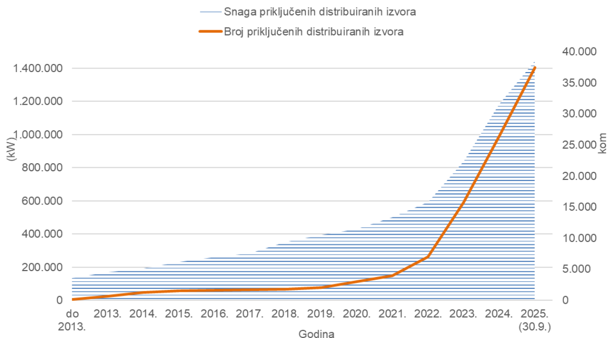
Slika 4-9 Porast broja i snage priključenih distribuiranih izvora u razdoblju od 2013. do 30.9.2025. godine
