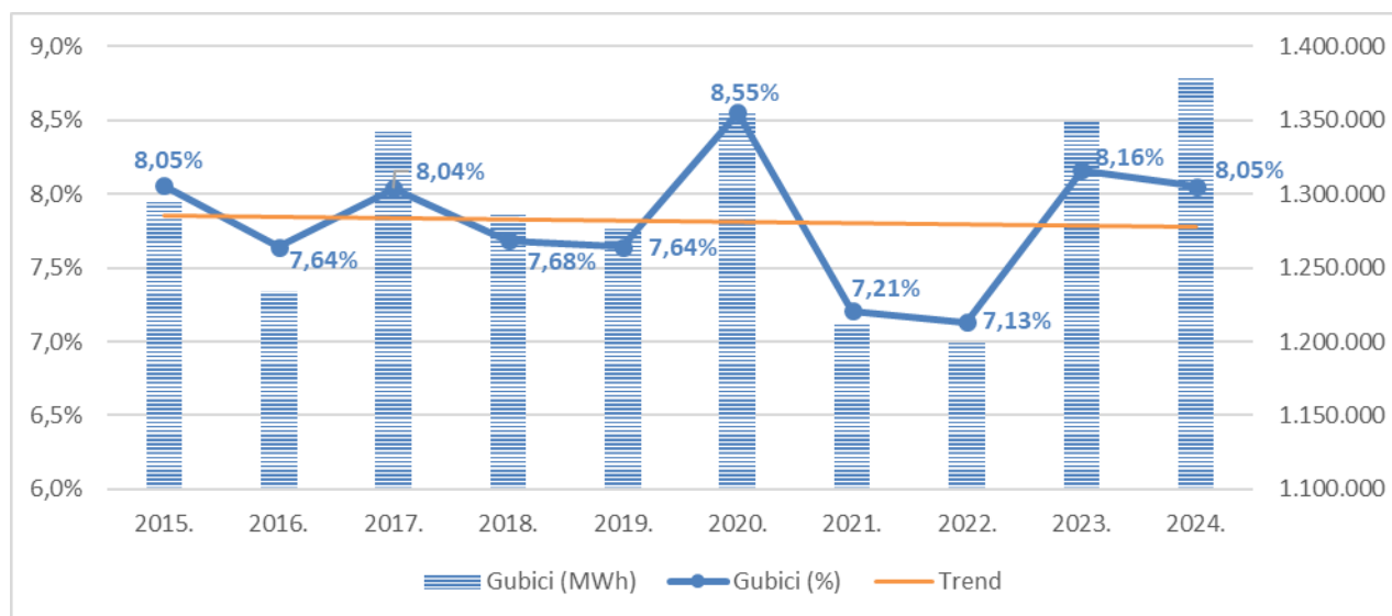
Slika 4-3 Gubici električne energije u razdoblju 2015. – 2024.
