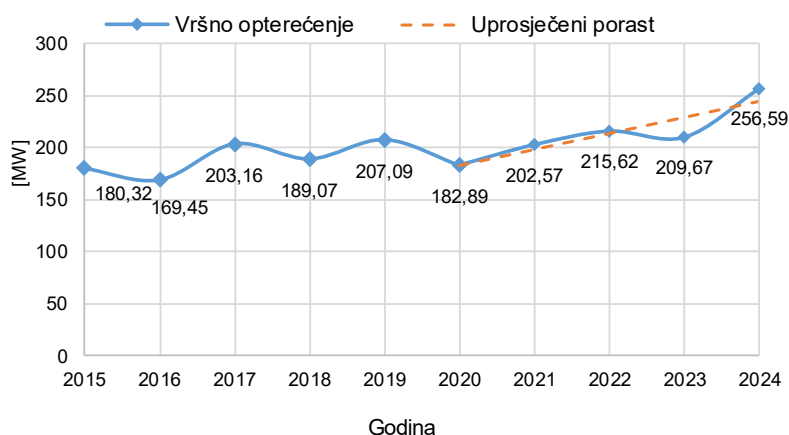
Ostvarena vršna opterećenja u razdoblju 2015. – 2024.
