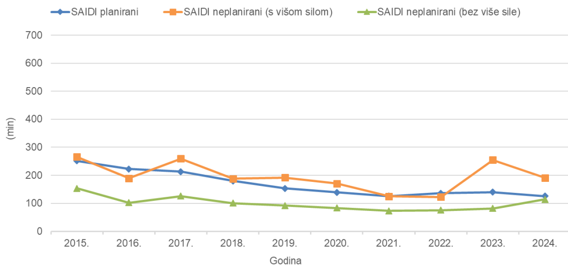
Slika 4-5 Prosječno trajanje dugotrajnih prekida napajanja svakog korisnika mreže (SAIDI) u razdoblju 2015. – 2024.
