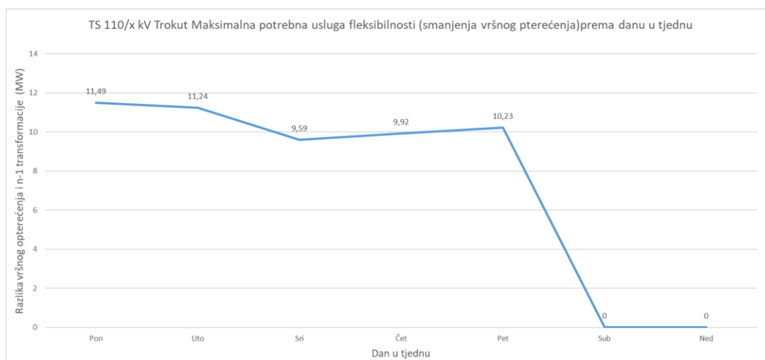
Slika 5-7 TS T110/x kV Trokut (DP Elektra Čakovec) – Maksimalna potrebna usluga fleksibilnosti (smanjenje vršnog opterećenja ) prema danu u tjednu (2023.g.)
