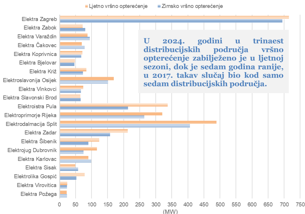
Slika 4-2 Zimsko i ljetno vršno opterećenje distribucijskih područja u 2024. godini
