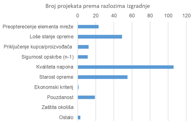
Slika 6-7 Razdioba planiranih ulaganja u izgradnju novih vodova 0,4 kV prema razlozima izgradnje (za razdoblje 2026. – 2028.)
