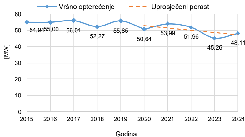
Ostvarena vršna opterećenja u razdoblju 2015. – 2024.
