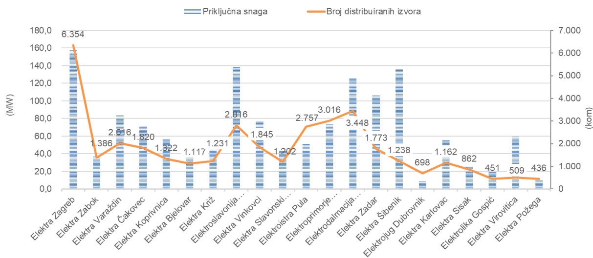
Slika 4-8 Priključna snaga i broj priključenih elektrana po distribucijskim područjima
