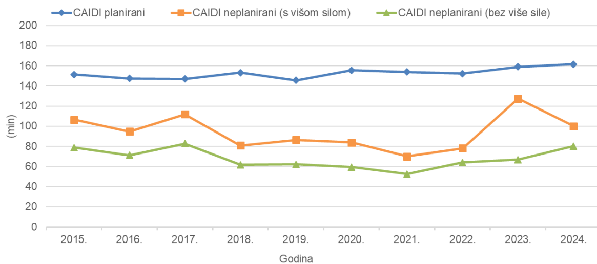
Slika 4-6 Prosječno trajanje dugotrajnih prekida napajanja po korisniku mreže (CAIDI) u razdoblju 2015. – 2024.
