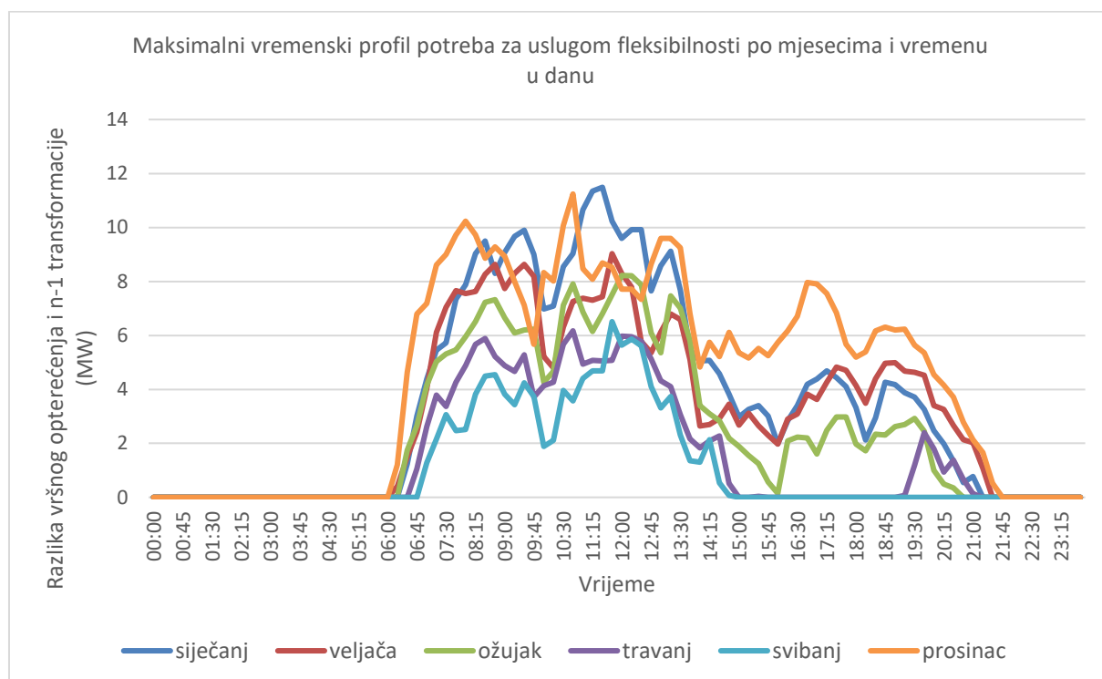
Slika 5-9 Maksimalna potrebna usluga fleksibilnosti (smanjenje vršnog opterećenja ) po mjesecima i vremenu u danu (2023.g.)
