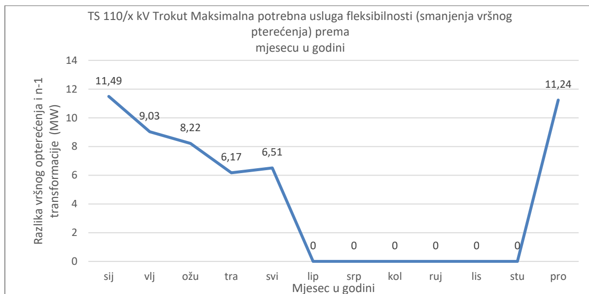
Slika 5-8 Maksimalna potrebna usluga fleksibilnosti (smanjenje vršnog opterećenja ) prema mjesecu u godini (2023.g.)
