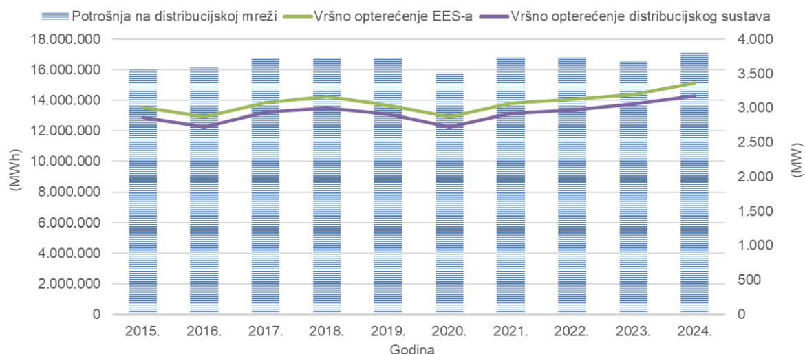
Slika 2 Vršno opterećenje EES-a i godišnja potrošnja električne energije na distribucijskoj mreži HEP ODS-a u razdoblju 2015. – 2024.
