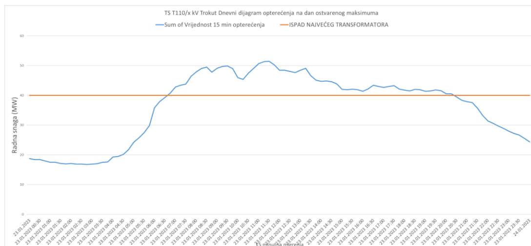
Slika 5-6 TS T110/x kV Trokut (DP Elektra Čakovec) – Dnevni dijagram opterećenja na dan ostvarenog maksimalnog opterećenja (2023.g.)
