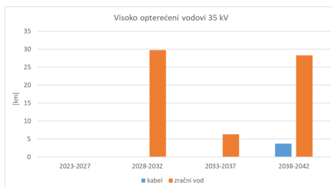
Slika 5-18 Duljina potrebnih novih 35 kV vodova
