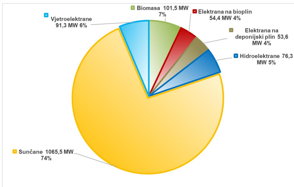
Slika 4-7 Priključna snaga po vrstama elektrana priključenih na distribucijsku mrežu
