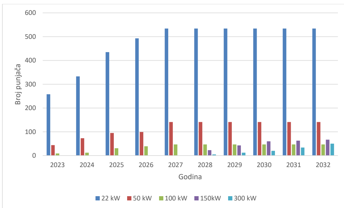
Slika 5-10 Projekcija broja punionica po godinama
