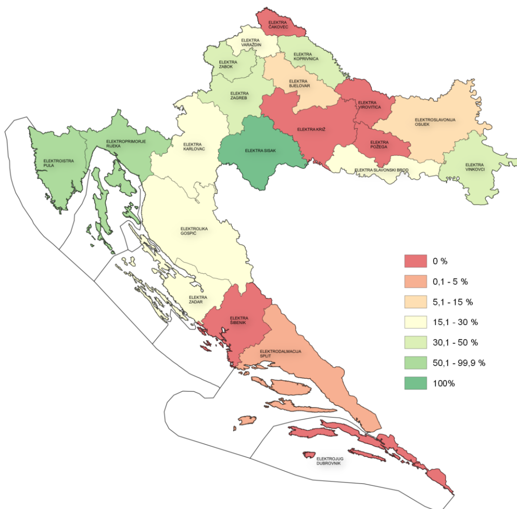
Slika 6-14 Pregled udjela TS SN/NN u pogonu na 20 kV po distribucijskim područjima
