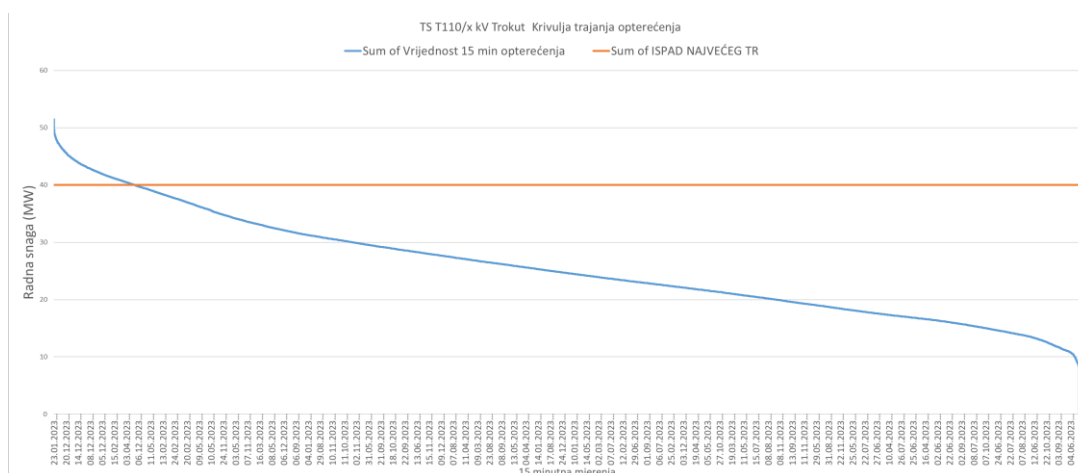
Slika 5-5 TS T110/x kV Trokut (DP Elektra Čakovec) - Krivulja trajanja opterećenja (2023.g.)
