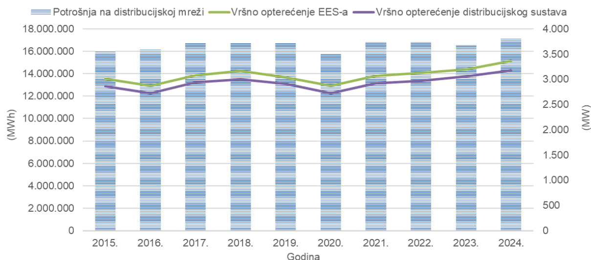
Slika 4-1 Vršno opterećenje EES-a i godišnja potrošnja električne energije na distribucijskoj mreži HEP ODS-a u razdoblju 2015. – 2024.
