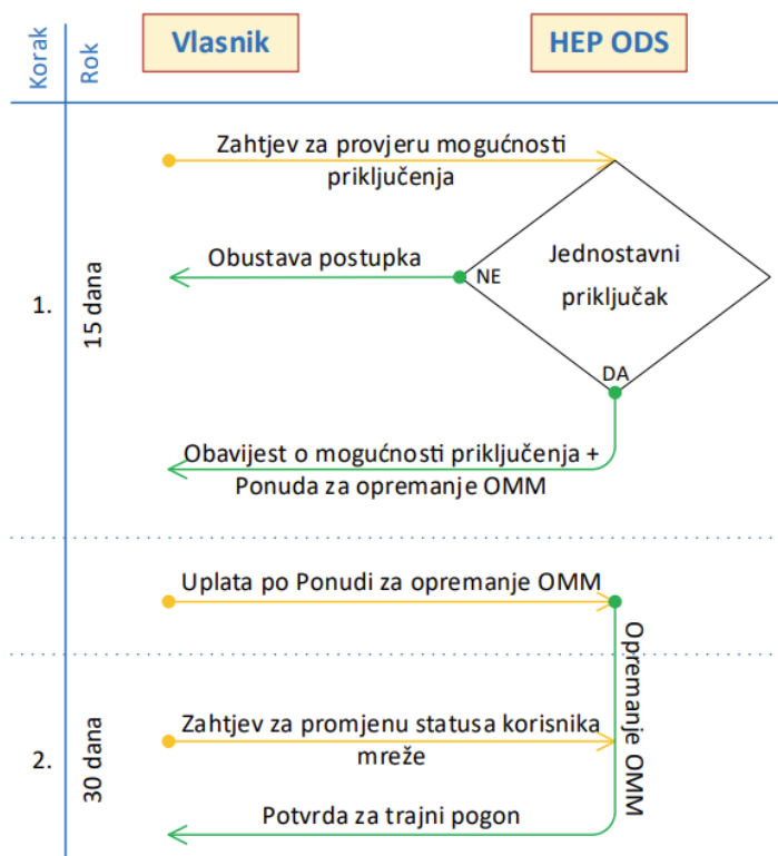
Slika 18 Postupak priključenja proizvodnog postrojenja na instalaciju postojećeg krajnjeg kupca priključne snage do uključivo 50 kW [46]
