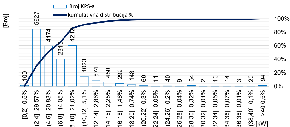
Slika 3 Statistička razdioba priključnih snaga u smjeru predaje električne energije u mrežu KPSO-a u RH na kraju 2024. godine [43]
