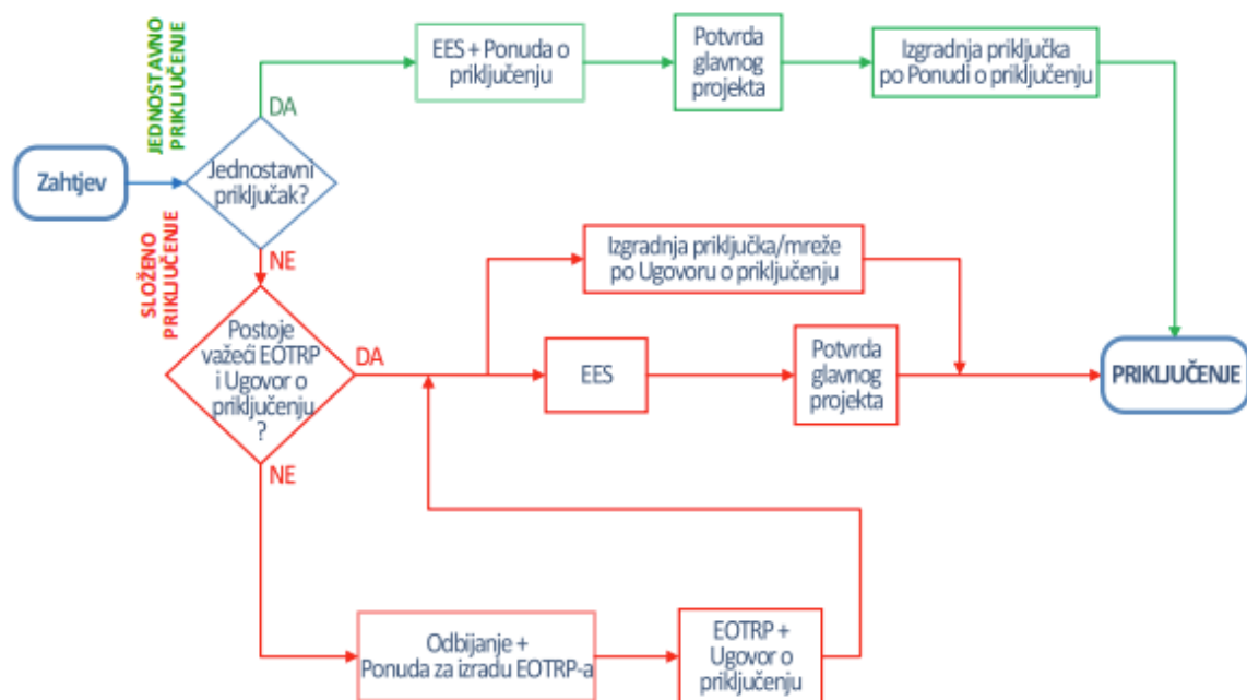
Slika 19 Načelna shema vrsta postupaka priključenja za krajnje kupce i KKVP-e [46]
