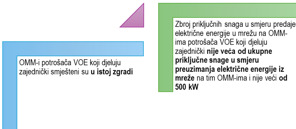
Slika 14 Uvjeti pod kojima su opskrbljivači električne energije dužni otkupljivati povremene viškove električne energije od potrošača VOE koji djeluju zajednički (SPVOE) i koji su uredili dijeljenje električne energije
