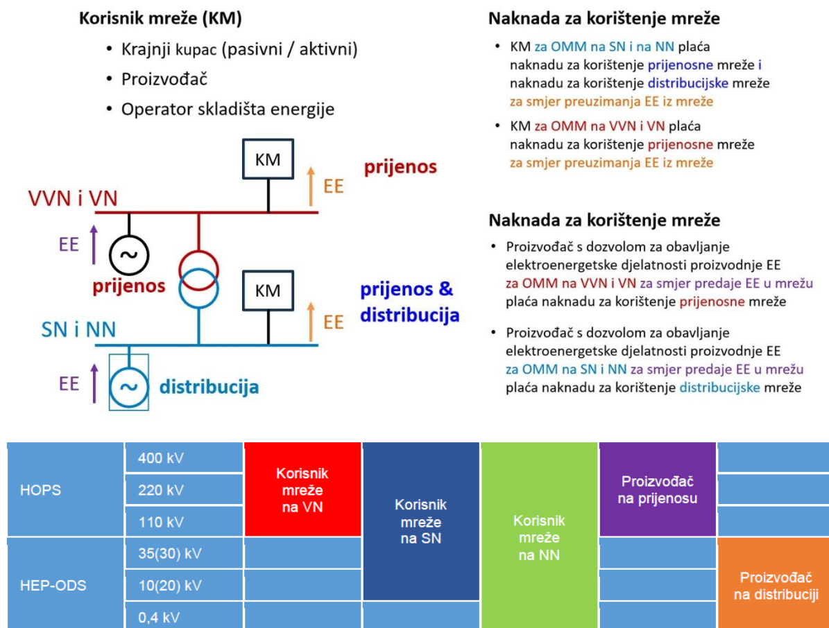
Slika 46 Plaćanje naknade za korištenje mreže u ovisnosti o smjeru toka EE (preuzimanje EE iz mreže i predaja EE u mrežu) te naponskoj razini na kojoj se nalazi OMM (VN – visoki i vrlo visoki napon, SN – srednji napon, NN – niski napon)
