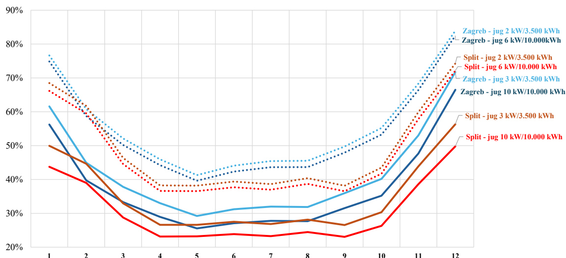
Slika 23 Primjeri udjela samoopskrbe po mjesecima PVOE-a - KPSO-a iz kategorije kućanstvo s godišnjom potrošnjom 3.500 kWh i 10.000 kWh i SE snage 2, 3, 6 i 10 kW s orijentacijom prema jugu u Zagrebu i Splitu
