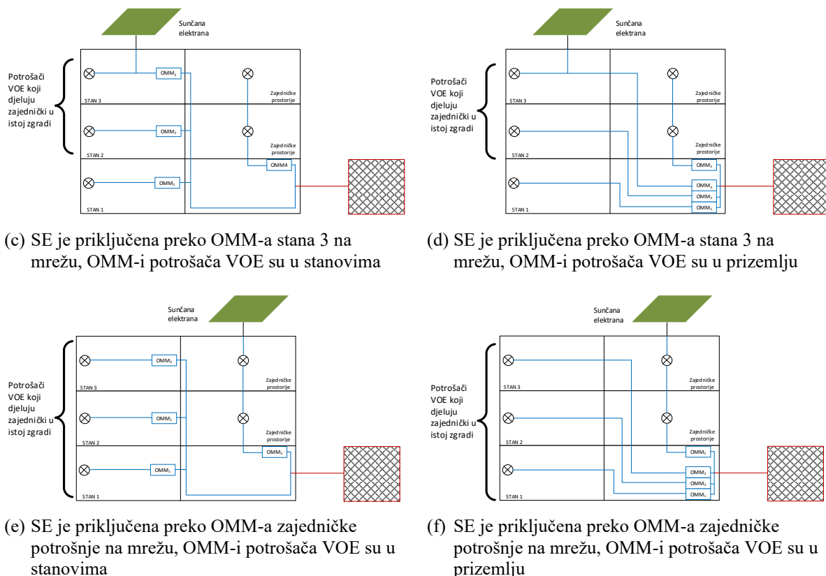
Slika 13 Varijante potrošača VOE koji djeluju zajednički (SPVOE)
