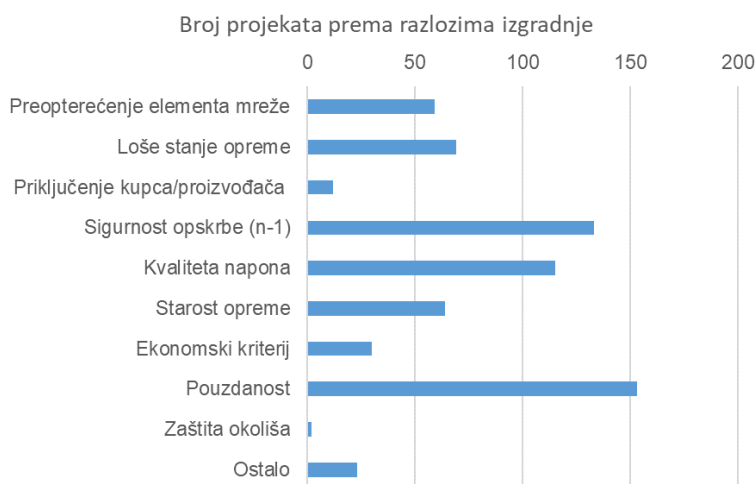
Slika 6-5 Razdioba planiranih ulaganja u izgradnju novih vodova 10(20) kV prema razlozima izgradnje (za razdoblje 2027. – 2029.)
