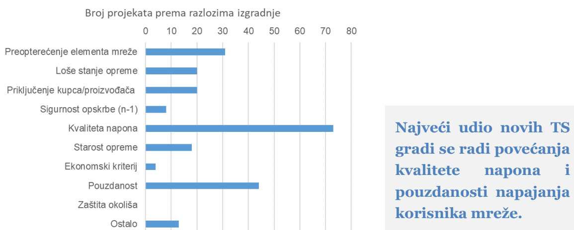
Slika 6-3 Razdioba planiranih ulaganja u izgradnji novih RS 10(20) kV i TS 10(20)/0,4 kV prema razlozima izgradnje (za razdoblje 2027. – 2029.)
