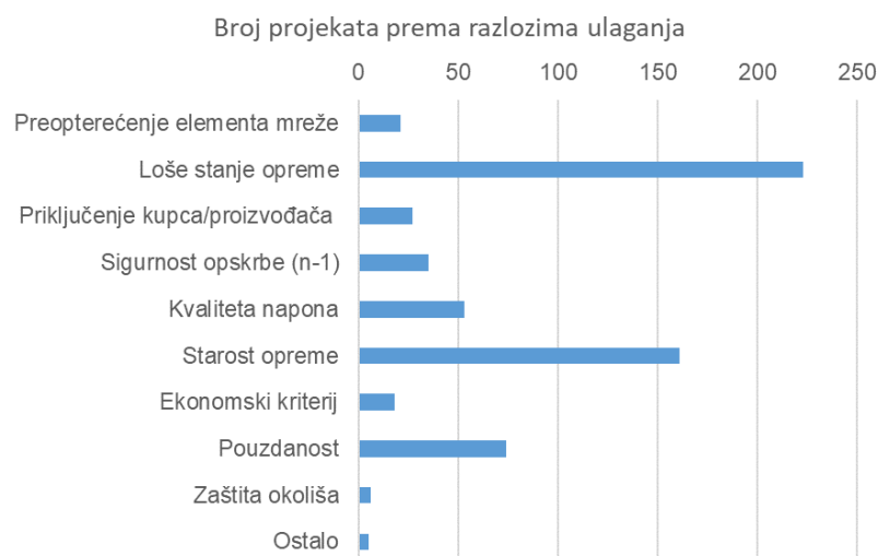
Slika 6-4 Razdioba planiranih ulaganja u rekonstrukcije i revitalizacije RS 10(20) kV i TS 10(20)/0,4 kV prema razlozima izgradnje (za razdoblje 2027. – 2029.)
