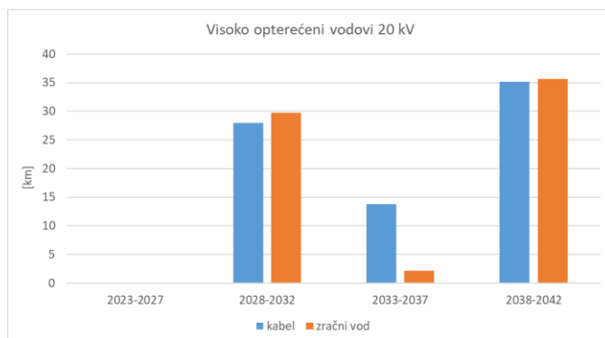
Slika 5-19 Duljina potrebnih novih 20 kV vodova
