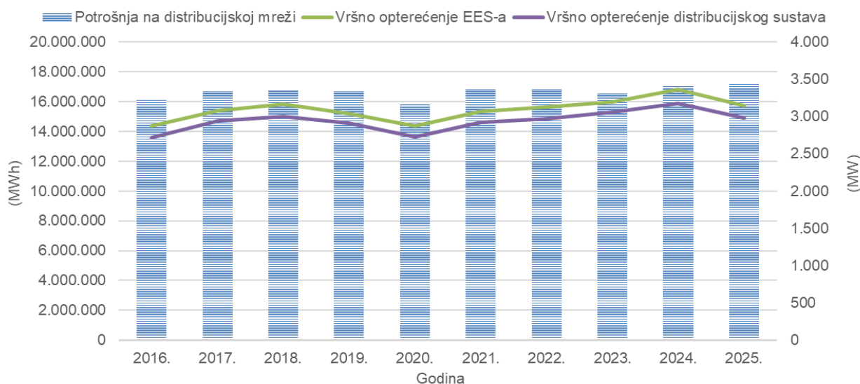
Slika 4-1 Vršno opterećenje EES-a i godišnja potrošnja električne energije na distribucijskoj mreži HEP ODS-a u razdoblju 2016. – 2025.
