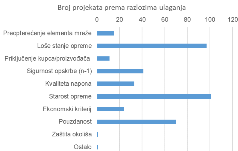
Slika 6-6 Razdioba planiranih ulaganja u rekonstrukcije i revitalizacije vodova 10(20) kV prema razlozima izgradnje (za razdoblje 2027. – 2029.)
