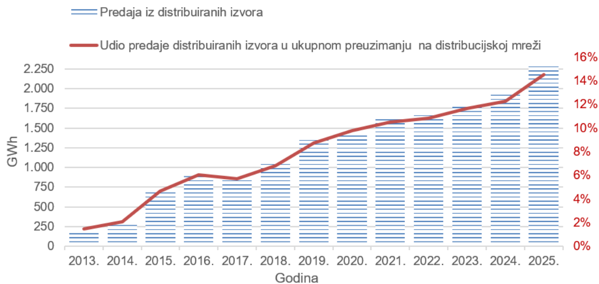
Slika 4-11 Godišnja predaja električne energije iz distribuiranih izvora
