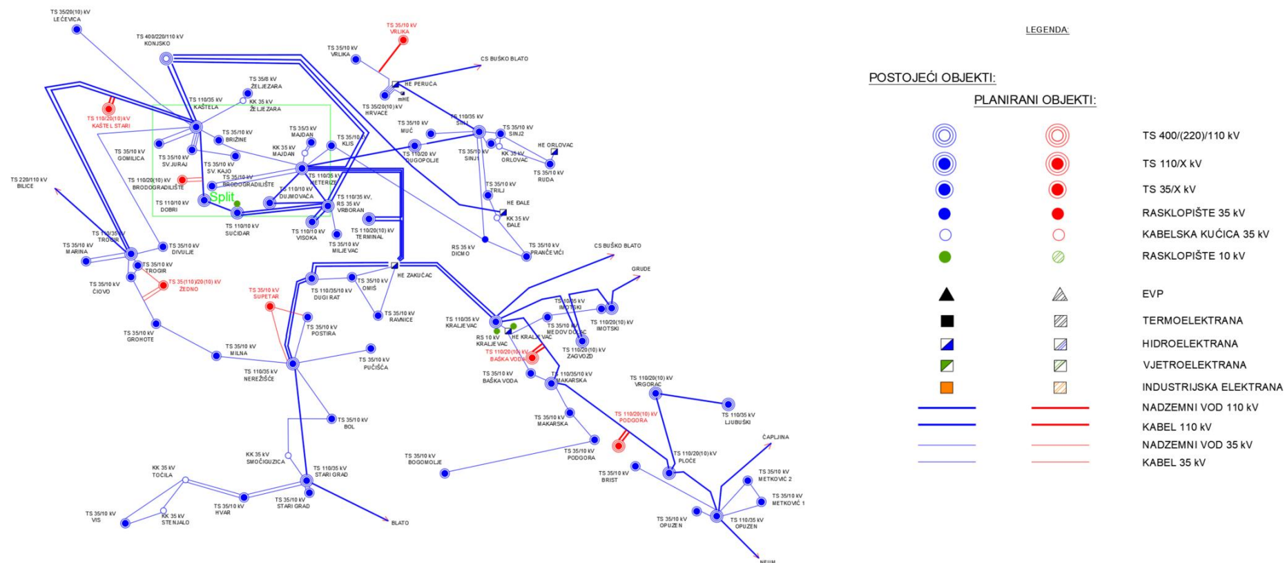
Slika 1. Shematski prikaz 110 kV i 30(35) kV mreže distribucijskog područja
