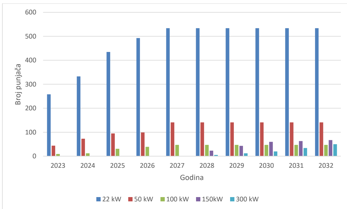
Slika 5-10 Projekcija broja punionica po godinama
