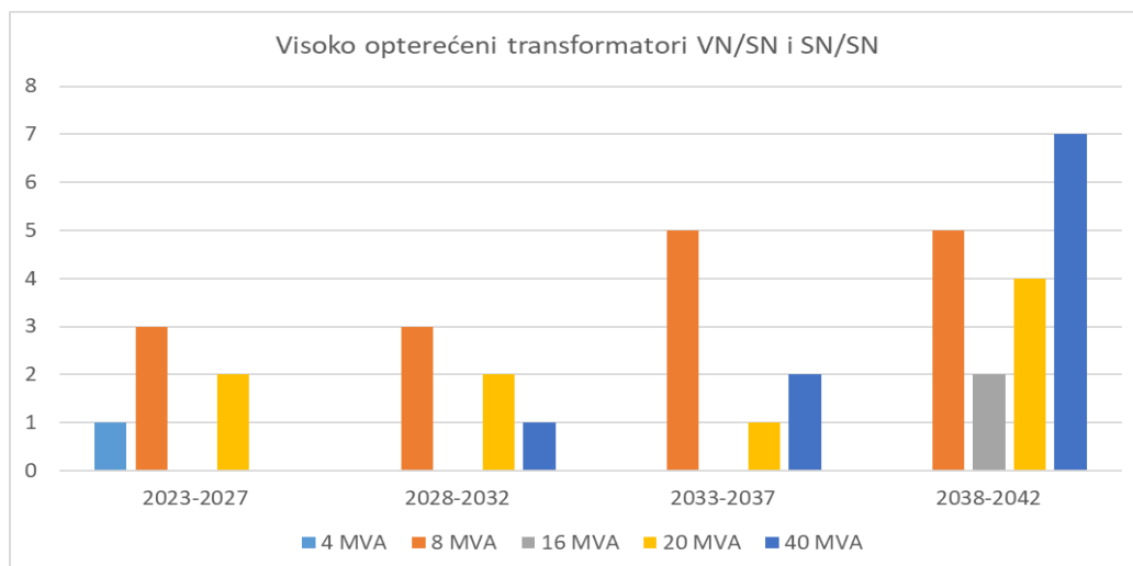
Slika 5-12 Broj potrebnih novih transformatora – Pojne točke
