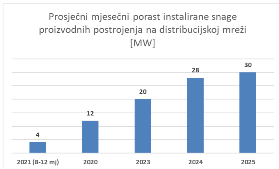
Slika 4-10 Trend porasta instalirane snage priključenih distribuiranih izvora
