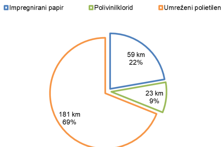
Slika 3-17 Prikaz udjela podmorskih kabela 10 kV i 20 kV po vrsti izolacije
