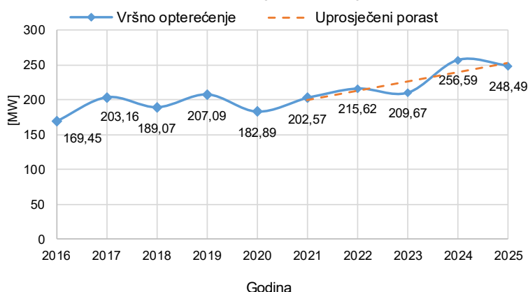
Ostvarena vršna opterećenja u razdoblju 2016. – 2025.
