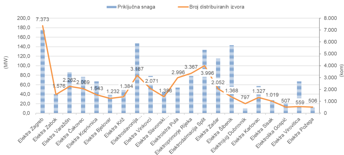
Slika 4-8 Priključna snaga i broj priključenih elektrana po distribucijskim područjima
