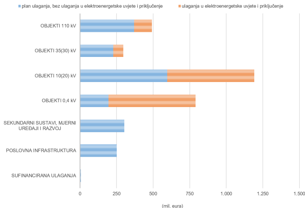
Slika 6-12 Pregled planiranih ulaganja u razdoblju 2027. – 2036. po vrstama ulaganja
