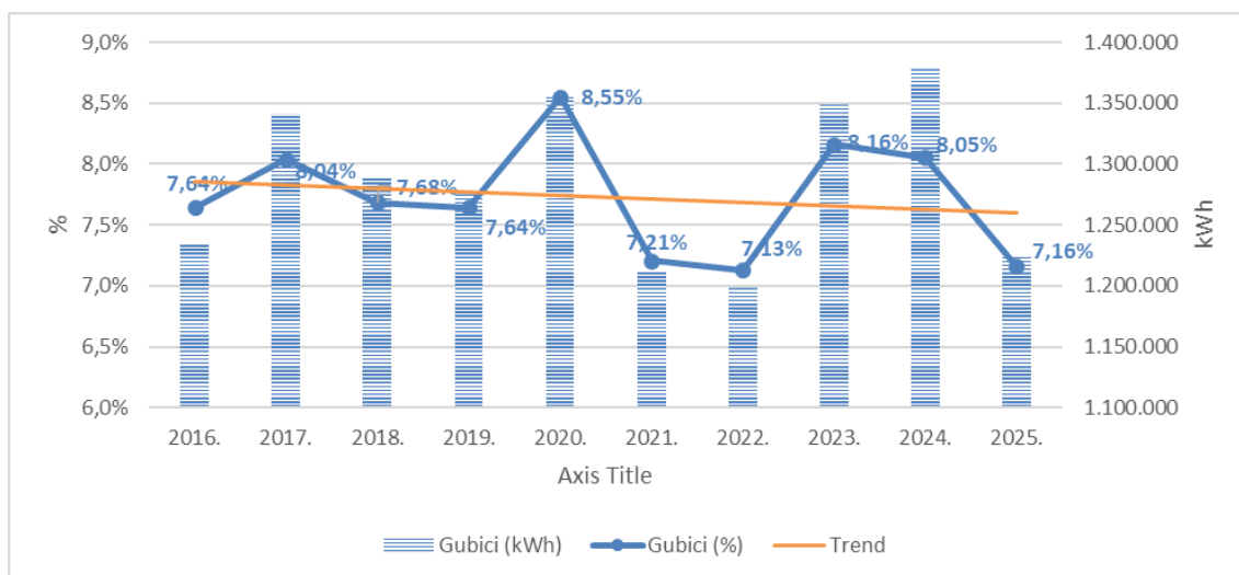
Slika 4-3 Gubici električne energije u razdoblju 2016. – 2025.
