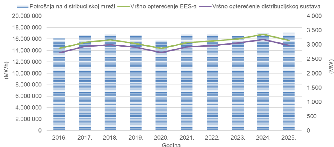
Slika 2 Vršno opterećenje EES-a i godišnja potrošnja električne energije na distribucijskoj mreži HEP ODS-a u razdoblju 2016. – 2025.
