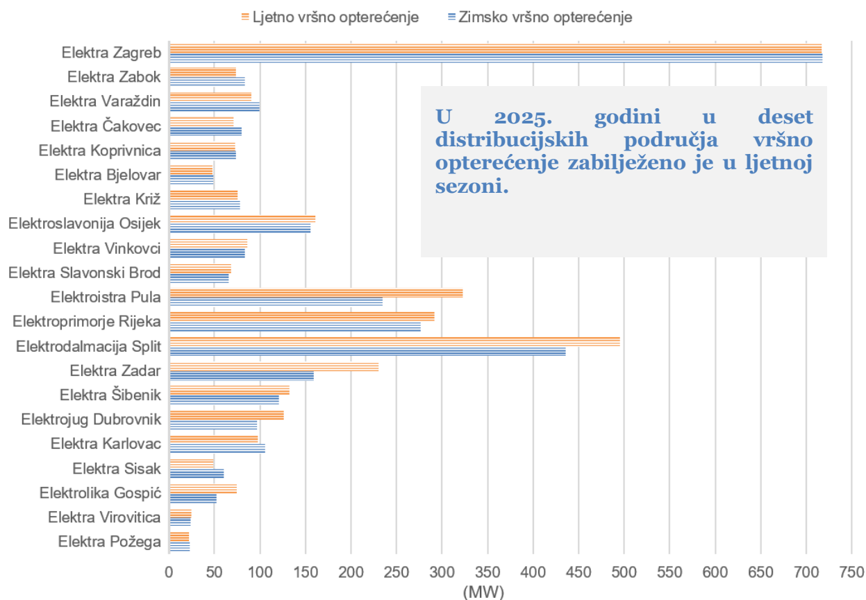
Slika 4-2 Zimsko i ljetno vršno opterećenje distribucijskih područja u 2025. godini
