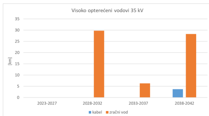
Slika 5-18 Duljina potrebnih novih 35 kV vodova
