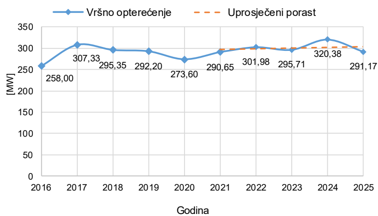
Ostvarena vršna opterećenja u razdoblju 2016. – 2025.
