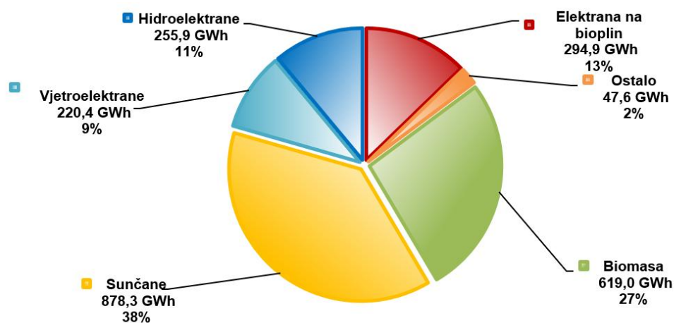
Slika 4-12 Godišnja predaja električne energije iz distribuiranih izvora po vrstama elektrana
