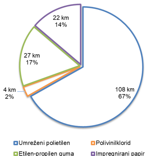
Slika 3-15 Duljine i udjeli podmorskih kabela 35 kV prema tehnološkoj izvedbi (izolaciji)
