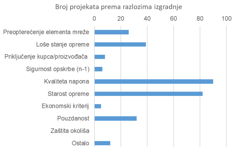
Slika 6-7 Razdioba planiranih ulaganja u izgradnju novih vodova 0,4 kV prema razlozima izgradnje (za razdoblje 2027. – 2029.)
