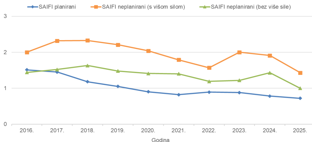
Slika 4-4 Prosječan broj dugotrajnih prekida napajanja svakog korisnika mreža (SAIFI) u razdoblju 2016. – 2025.
