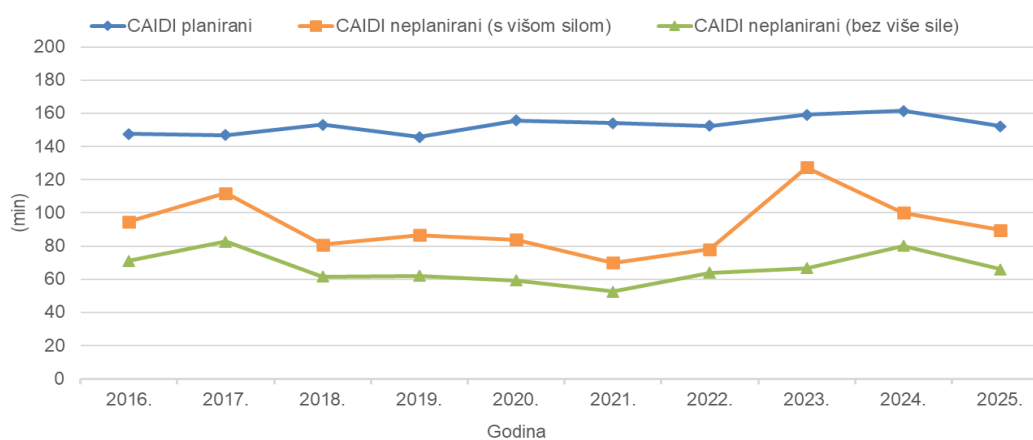
Slika 4-6 Prosječno trajanje dugotrajnih prekida napajanja po korisniku mreže (CAIDI) u razdoblju 2016. – 2025.
