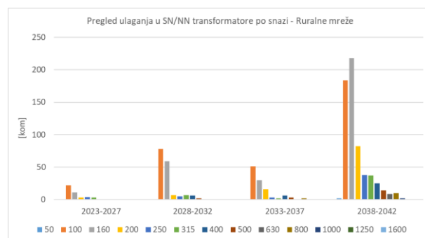
Slika 5-14 Broj potrebnih novih SN/NN transformatora za klaster Ruralne mreže
