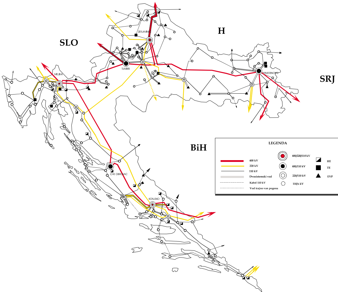
Slika 7. Prijenosna mreža na području Republike Hrvatske (stanje 2005. godine)
